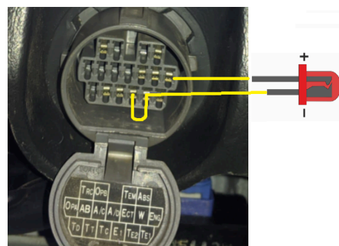
Рис.1с Перемычка + светодиод в DLC-2
