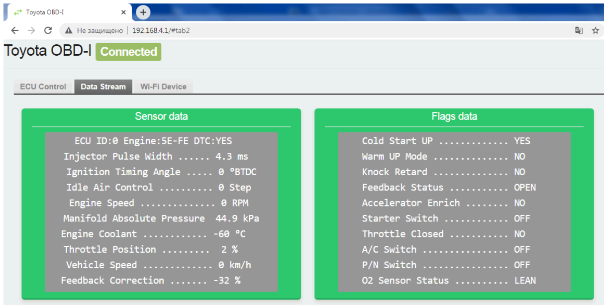
Рис.4 (Поток данных)
