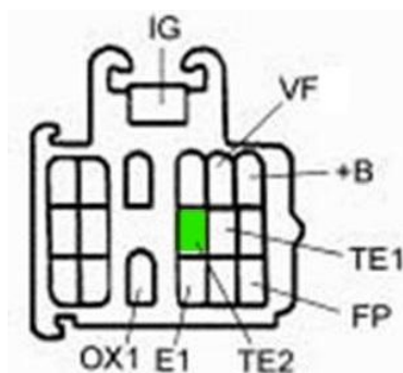
Рис.1а Разъем DLC-1 (17 Pin)
