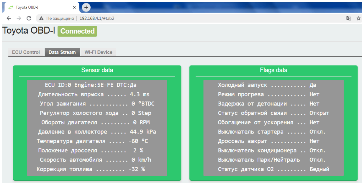
Рис.5 (Поток данных)
