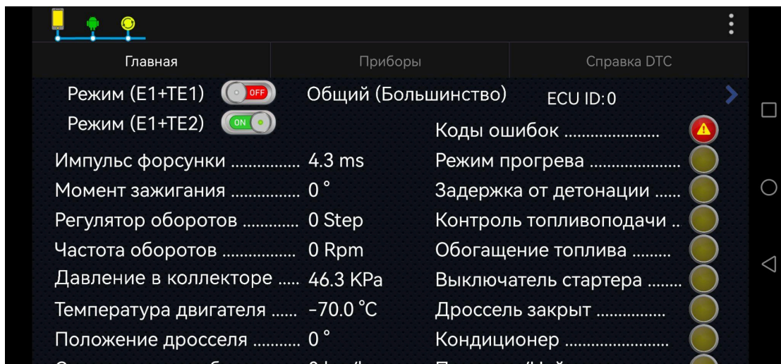
Рис.10 Режим чтения параметров проекта приложения Virtuino 6 Viewer
