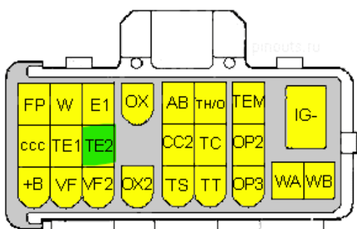
Рис.1б Разъем DLC-1 (23 Pin)
